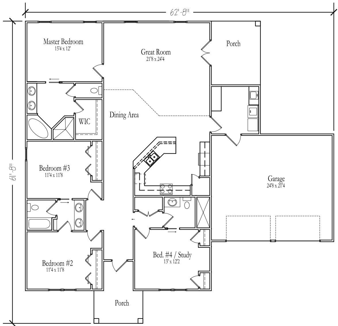
Floor Plan N.T.S
